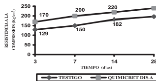
GRÁFICA DE RESISTENCIA A LA COMPRESIÓN CON 1.5% DE QUIMICRET DIS A
